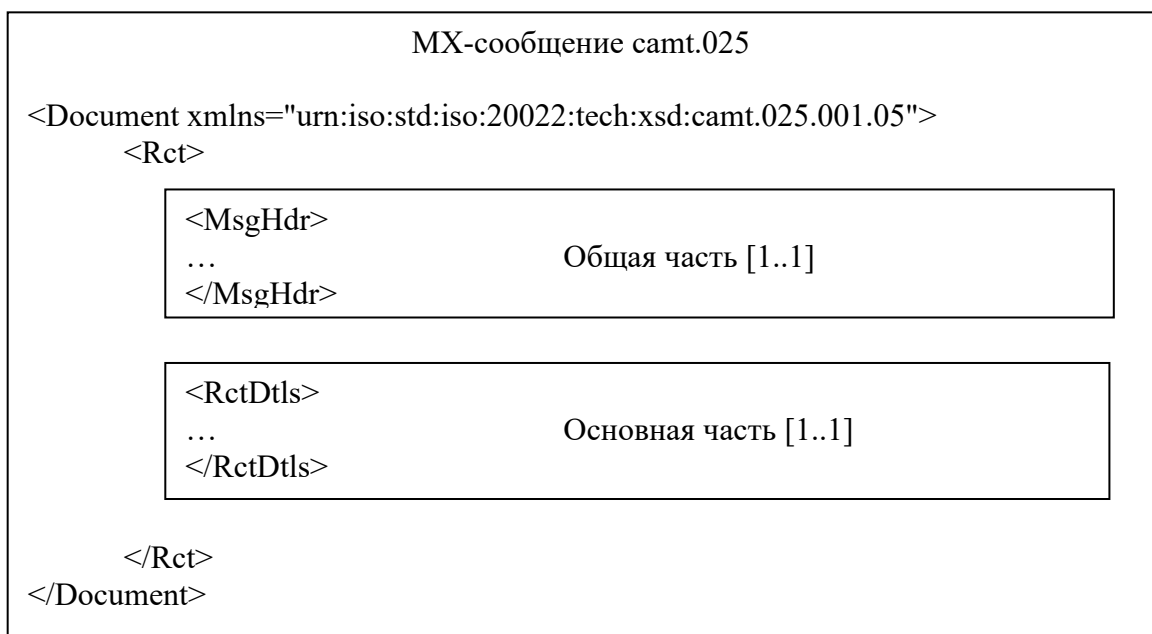
Рисунок 1 – Структура МХ-сообщения samt.025
